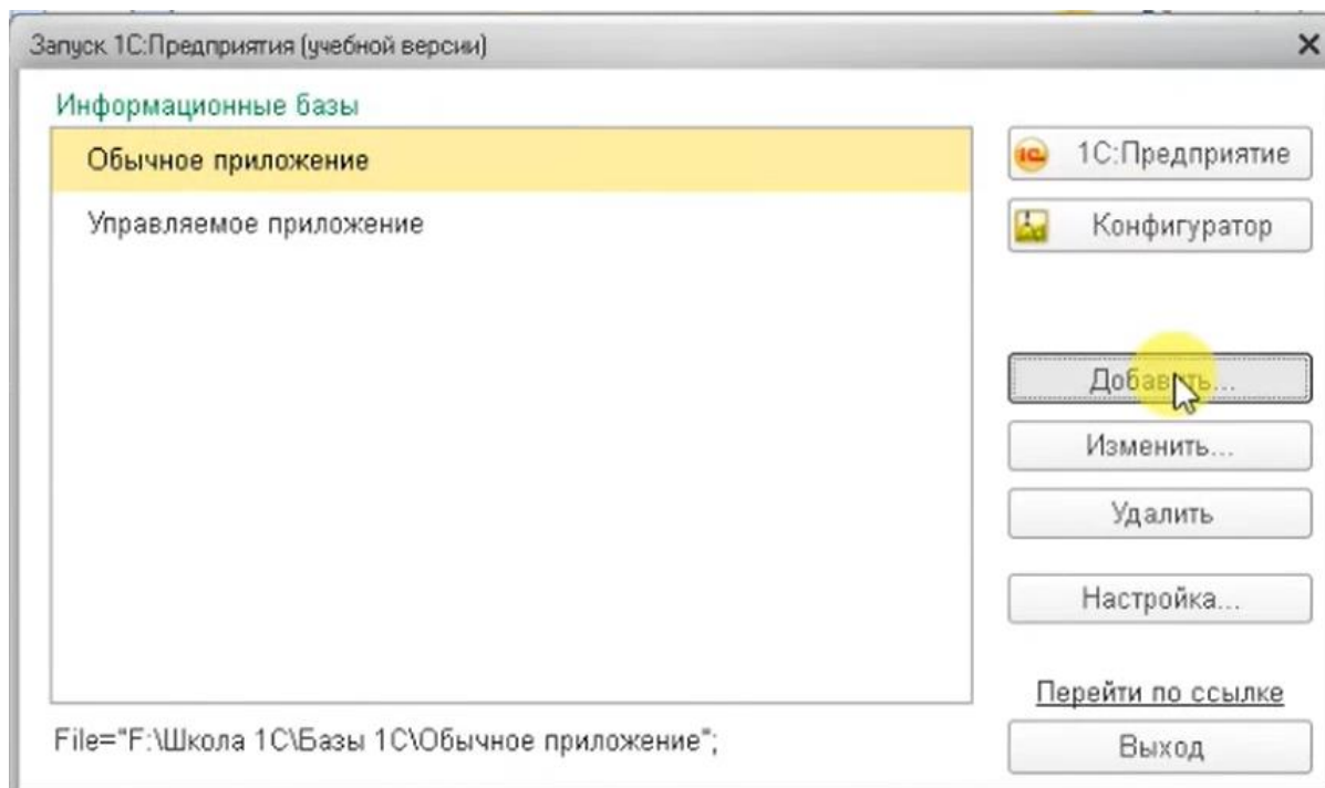
Рисунок 5 – Окно «Запуск»
