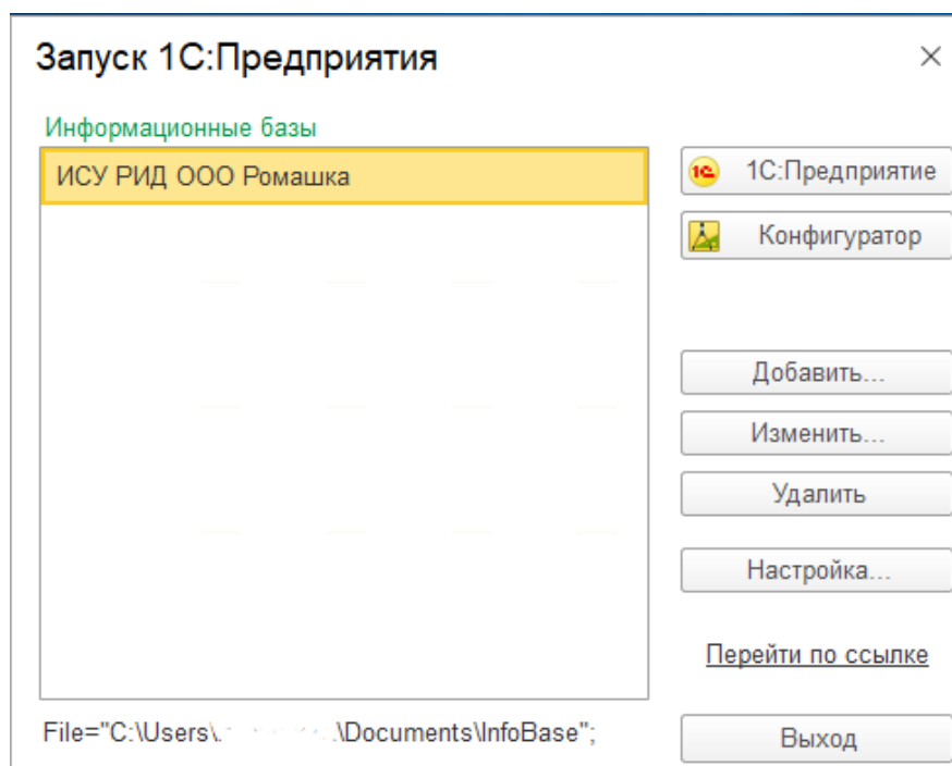
Рисунок 12 – Запуск «1С:Предприятие»
